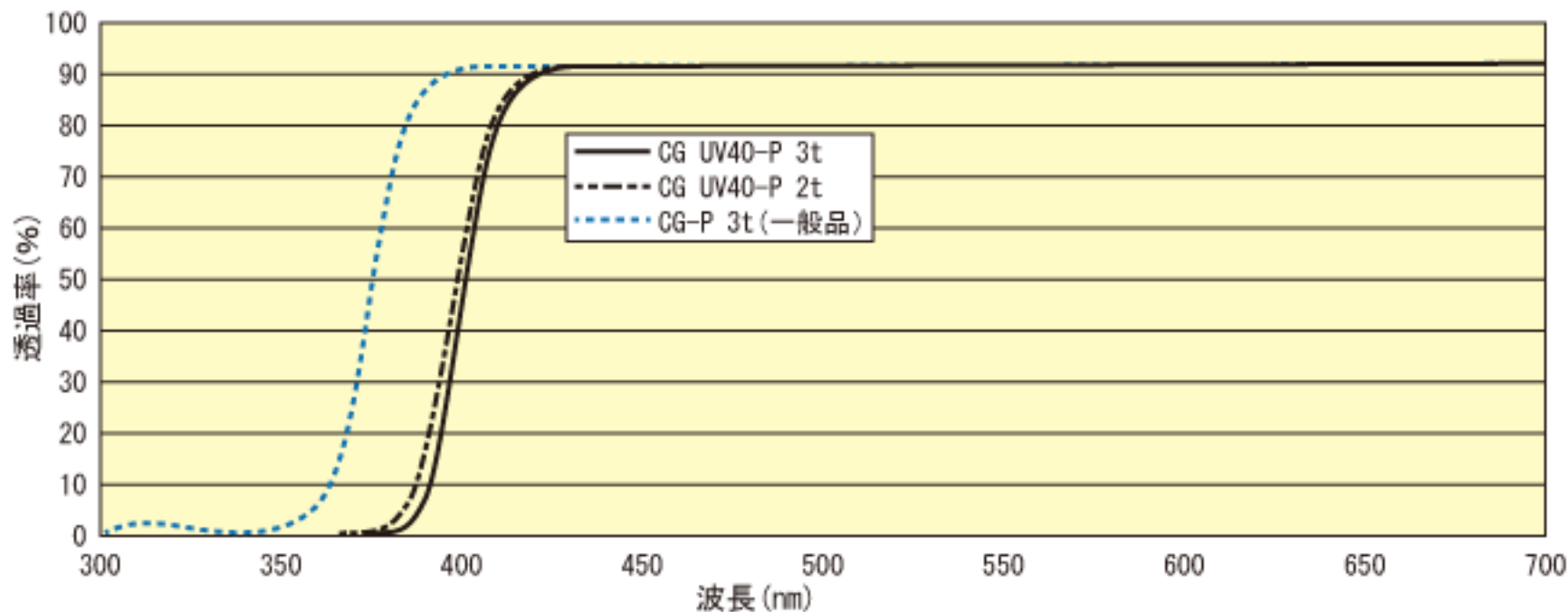
CGUV40板の全光線透過率と測色
